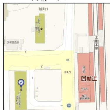
会場マップ
